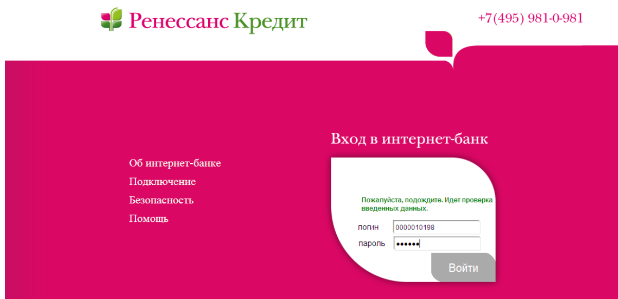
Рисунок 1.1. Аутентификация клиента
